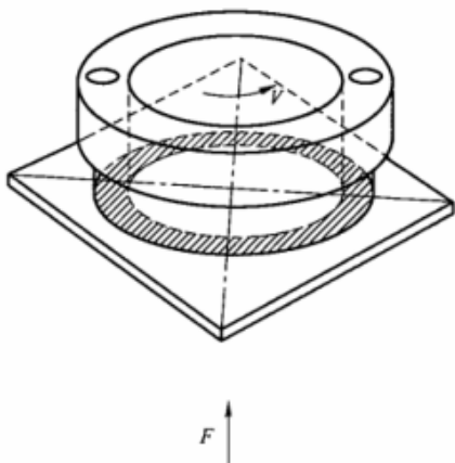
图3 端面摩擦磨损性能试验原理图
