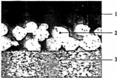
说明： 1——表面塑料层； 2——中间烧结层； 3——钢背层。 * 经供需双方协议，钢背层可采用铜镀层或无镀层。
