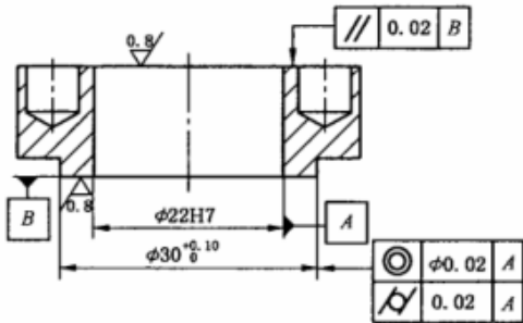
图5 对磨件几何精度要求
