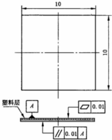
图 2 试样几何精度要求
